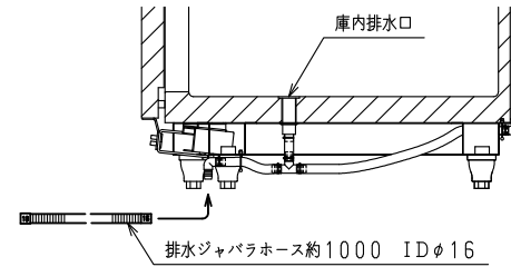
排水部詳細
