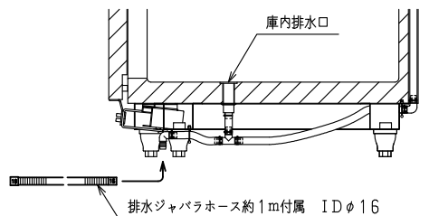
排水部詳細
