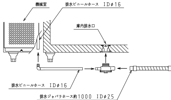
排水部詳細
