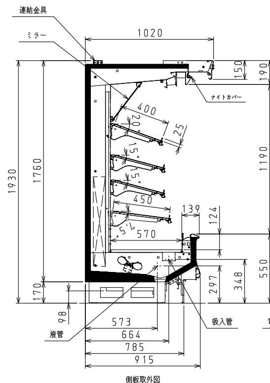
側板取外図
