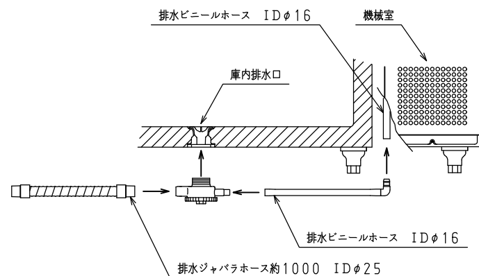
排水部詳細
